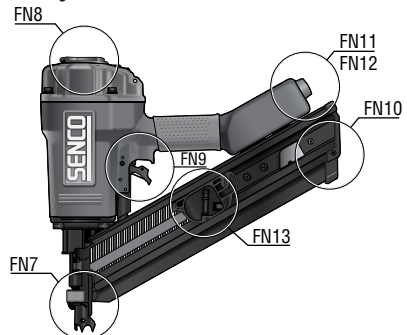
Rahmennagler
