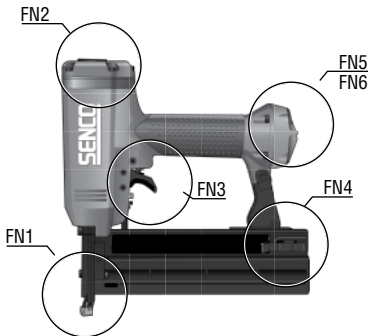
Stahlstiftnagler
